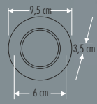
KN-05139 SPOT
