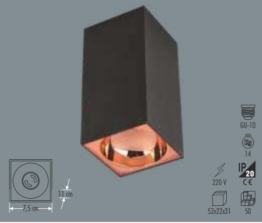
KN-05023 (SİYAH-PLATİN)
