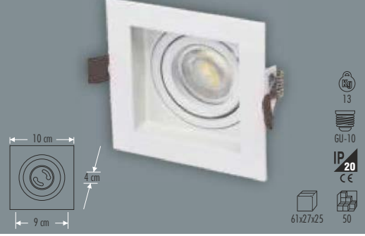
KN-05031 (BEYAZ-SİYAH)
