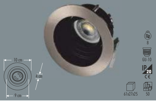
KN-05036 (SİYAH)
