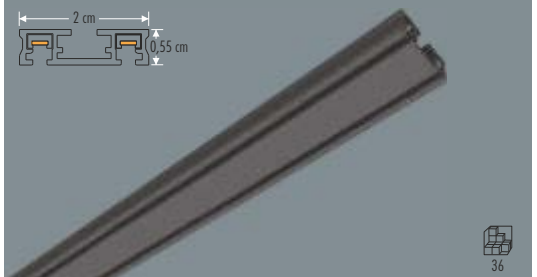
KN-05066 1 Metre ULTRA İNCE 0,55 cm KN-05067 2 Metre ULTRA İNCE 0,55 cm KN-05068 3 Metre ULTRA İNCE cm
