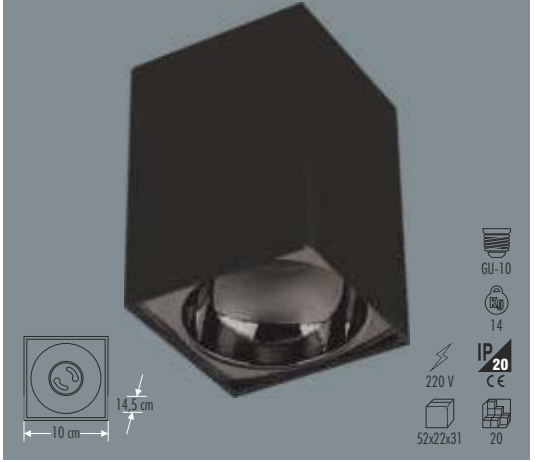
KN-05022 (SİYAH-PLATİN)
