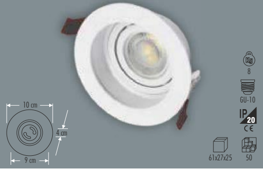
KN-05030 (BEYAZ-SİYAH)
