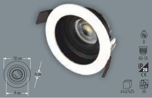
KN-05033 (SATIN-SİYAH)
